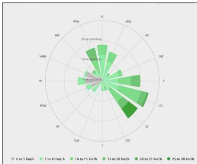
Obrázok 5 Veterná ružica
